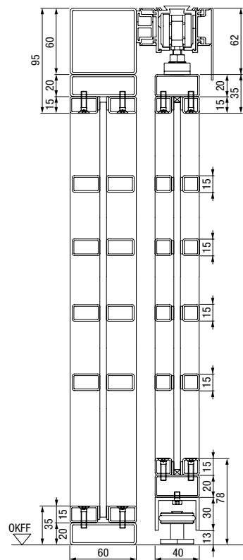
Vertikalschnitt 2-flügelige Stahl-Lofttür mit Seitenteil
