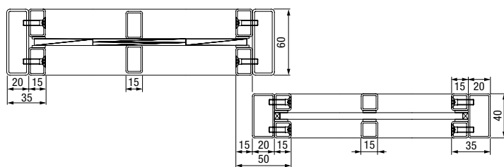
Horizontalschnitt 2-flügelige Stahl-Lofttür mit Seitenteil
