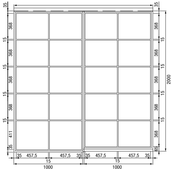
2-flügelige Stahl-Lofttür mit Seitenteil
